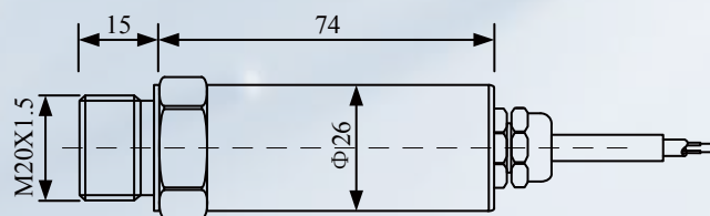
直接引线 (单位: mm)
