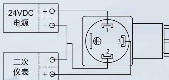
电压输出
