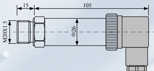
赫斯曼接头 (单位: mm)
